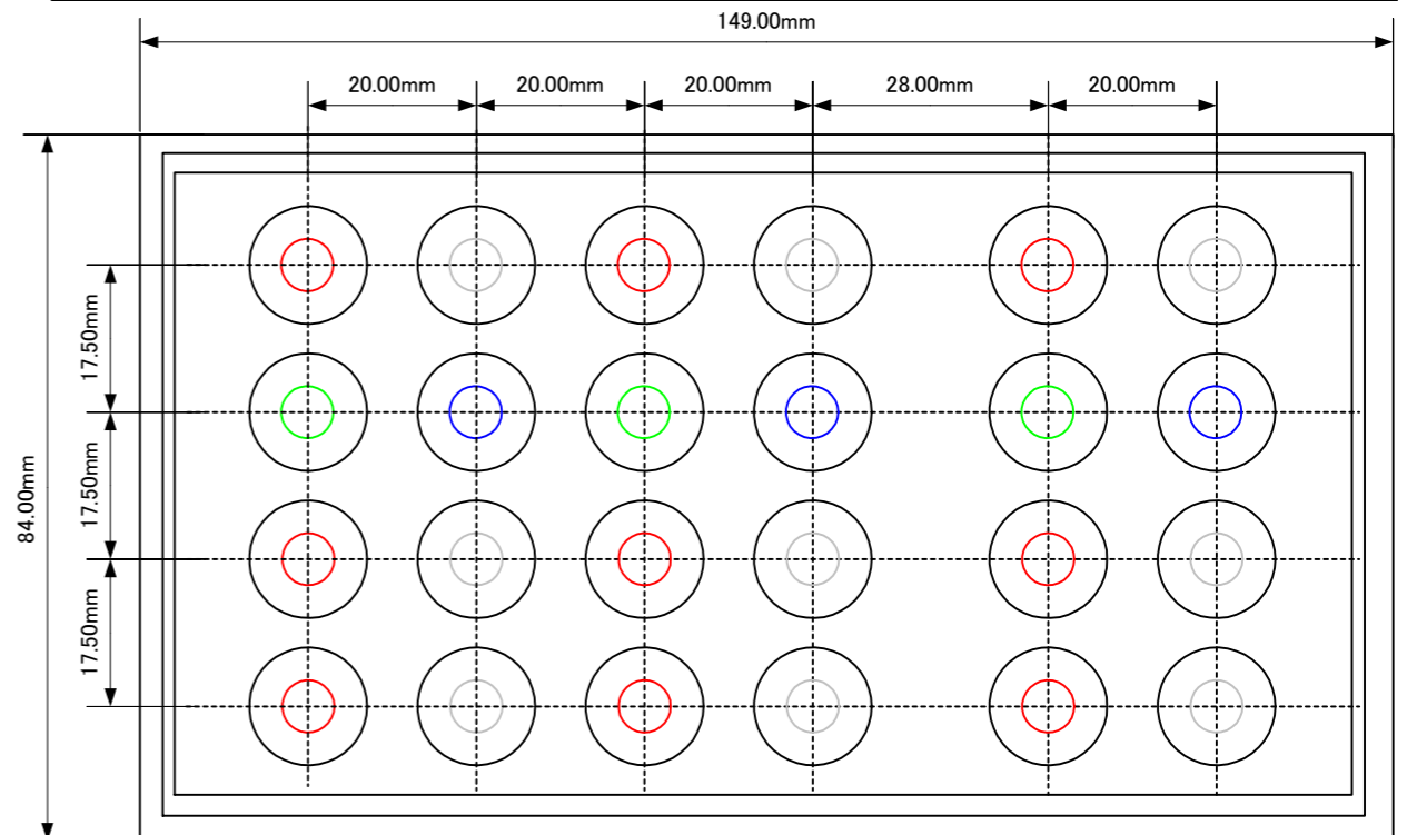
2系統 CH8-SEL2 WxHxD=149x84x170
